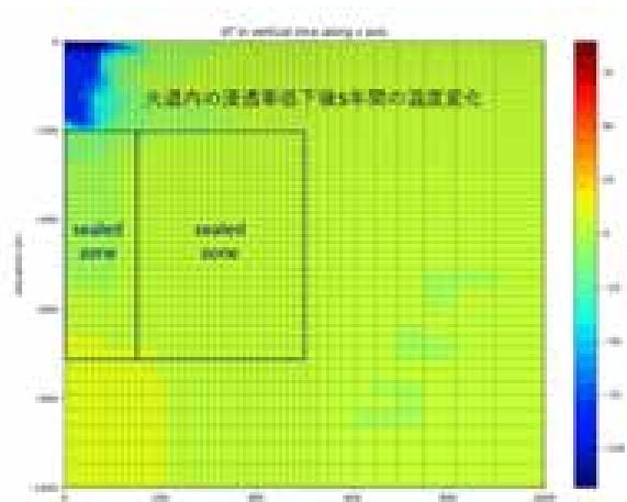
図 53. 浸透率低下後 5 年間の温度変化。
