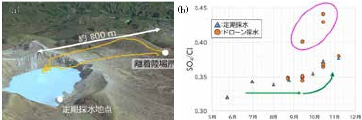
図 63. (a) 草津白根火山湯釜火口湖の湖底湧出孔付近、水深 20m からの採水。(b) 定点採水とドローン採水の比較。定点で SO_4/C1 比が長期的に上昇するよりも前に、ドローン採水では高い SO_4/C1 比が検出された。
