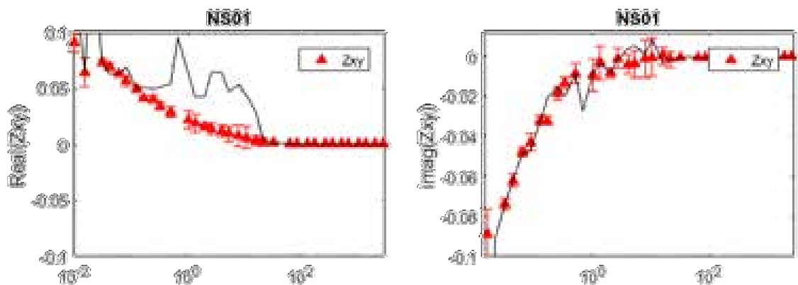
図 13. 改善された応答関数の例。黒線は以前の応答関数、赤線は再解析結果。
