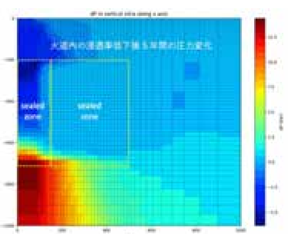
図 54. 浸透率低下後 5 年間の圧力変化。
