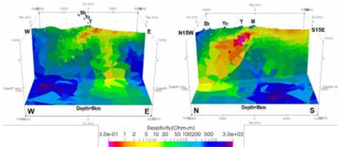
図 22. 草津白根火山周辺の暫定比抵抗構造モデル。左：本白根山山頂を通る東西断面。右：本白根山山頂を通る N15^{\circ} W-S15^{\circ} E 断面。海拔下 8km の水平断面も併せて表示している。Sh: 志賀山・鉢山、Yo: 横手山、Y: 湯釜、M: 本白根山。白点は MT 観測点。
