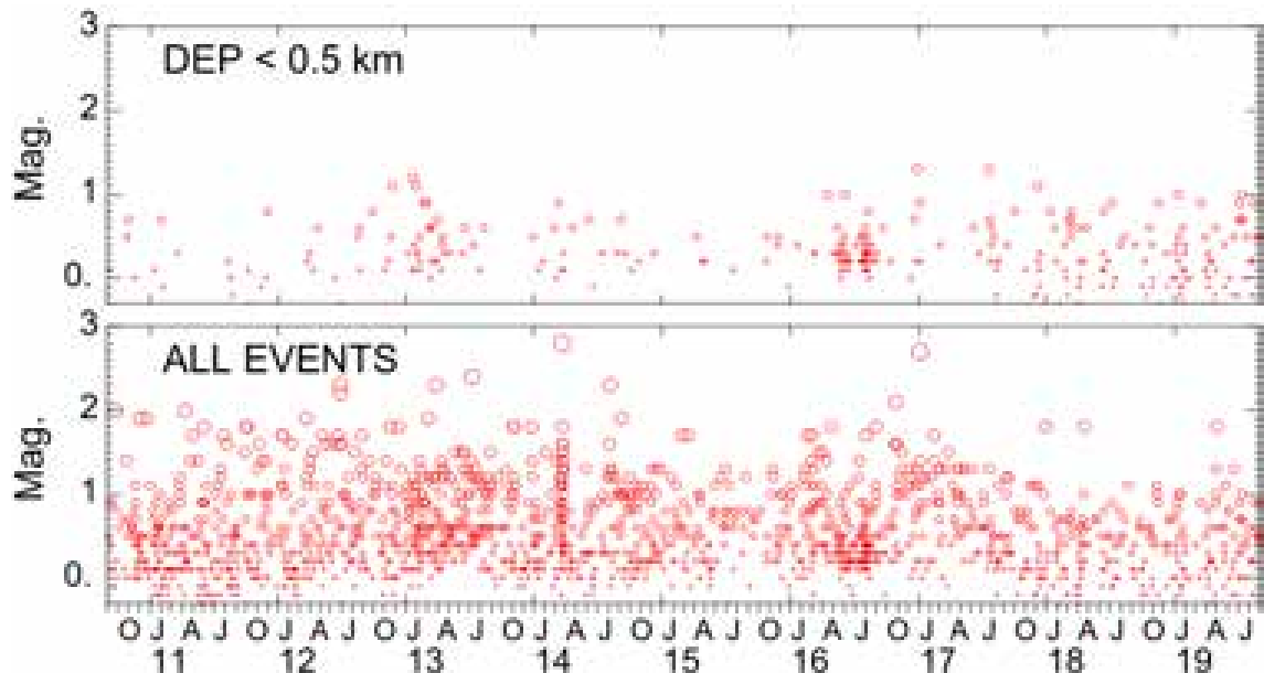
図7. 庁検出カタログを用いて震源再決定した地震のMT図。上：震源の深さ0.5 km以浅で発生した地震。下：すべての地震。
