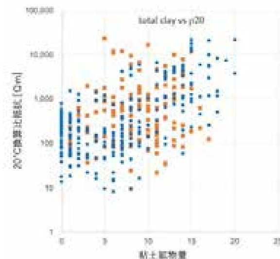
図 57. 粘土鉱物量と比抵抗の関係。
