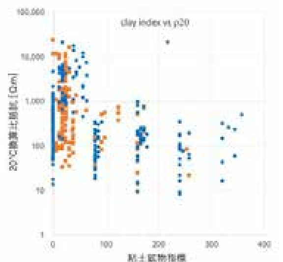
図 58. 粘土鉱物導電指標と比抵抗の関係。
