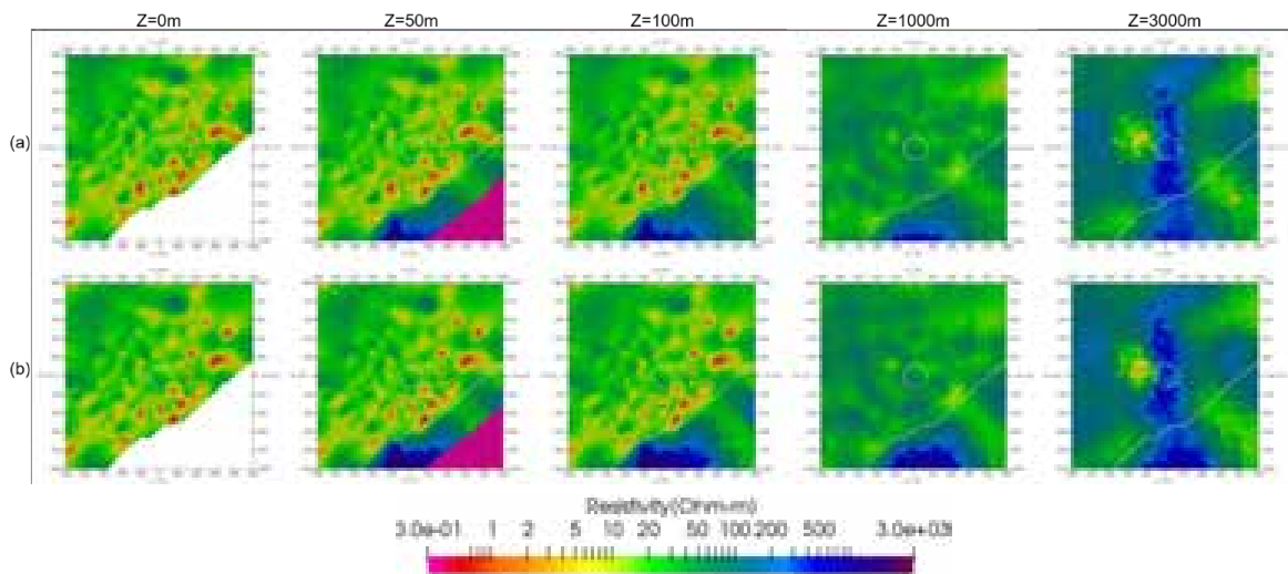
図 48. 倶多楽火山の 3 次元比抵抗構造モデル。中心から半径 15km の領域の海底地形に (a) M7006 データを用いた場合、(b) 周囲と同じ J-EGG500 データを用いた場合。両モデルとも、左から海抜下 0m、50m、100m、1000m、3000m の水平断面を示す。白線は倶多楽湖の輪郭および海岸線を表す。
