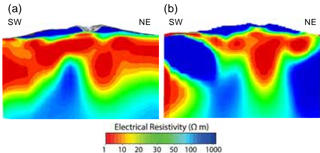
図 14. 三宅島の北東一南西断面の地下比抵抗構造。
