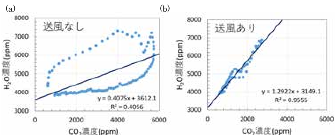
図 64. H_2O と CO_2 濃度比の測定。 H_2O と CO_2 濃度を同時測定し、同時刻における両ガスの濃度を表示したもの。センサ応答時間が一致しているとき、その直線的関係に基づき濃度比を見積もることができる。(左) 送風のない状態。(右) 送風を与えた場合。
