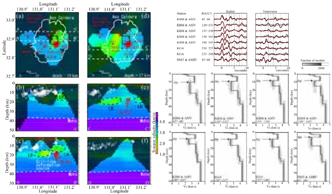
図 41. 阿蘇火山での解析例 (Abe et al., 2017 32) )。右図はレーシーバ関数とそれから得られた 1 次元速度構造の一部。多数得られる 1 次元構造から、それぞれの波線の位置を考慮することで左図のような 3 次元構造が推定できる。
