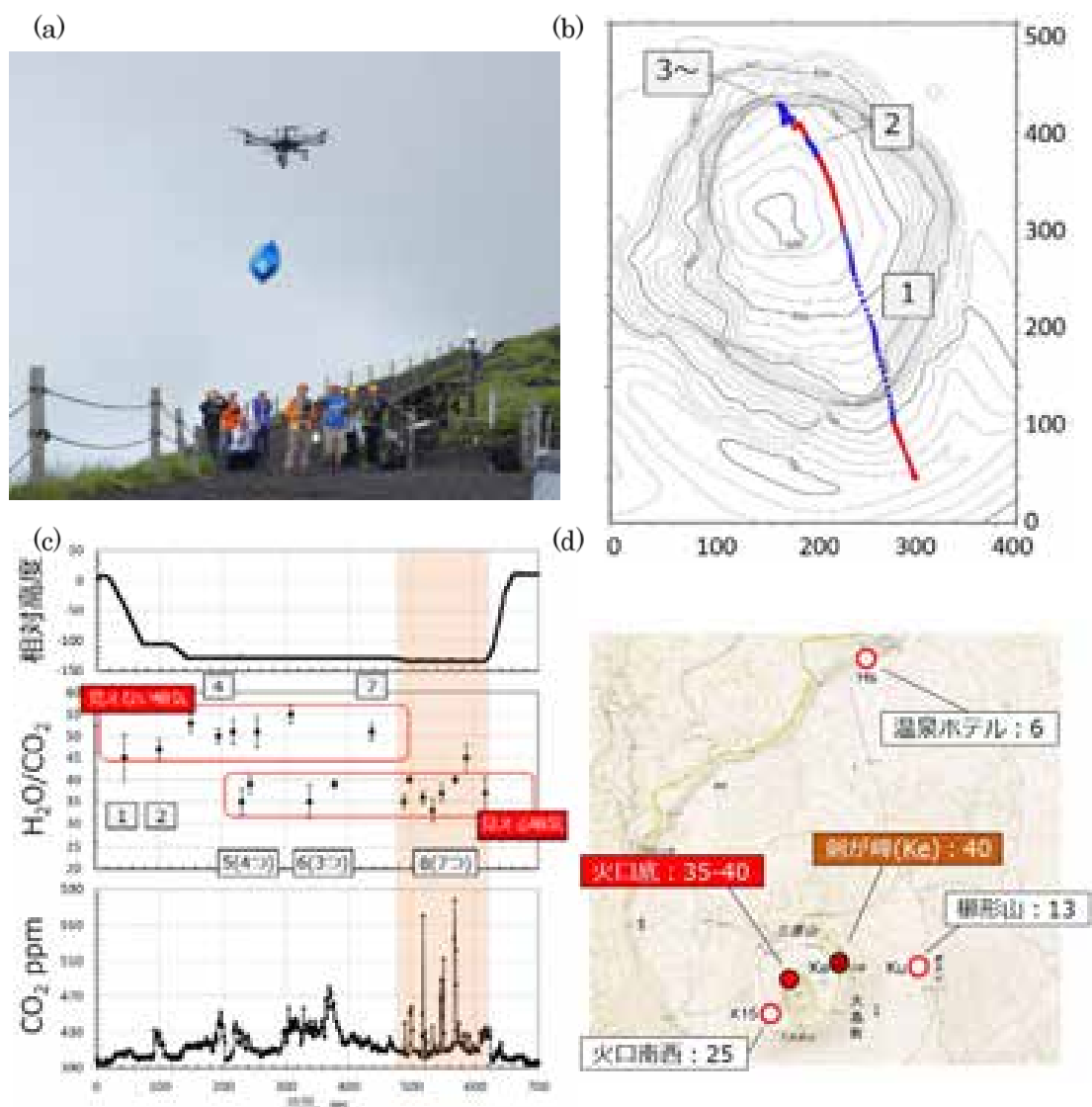
図 65. (a) 離陸の様子。三原新山展望台付近。(b) 飛行経路。青は火山ガスが計測された領域。(c) ドローン相対高度、見積もられた組成比、および処理前の測定 CO_2 濃度値。ピーク 1、2、4 および 7 は目に見えないが火口内に滞留している噴気ガス。オレンジハッチはウインチ降下中に対応する。(d) H_2O/CO_2 組成比の空間分布。
