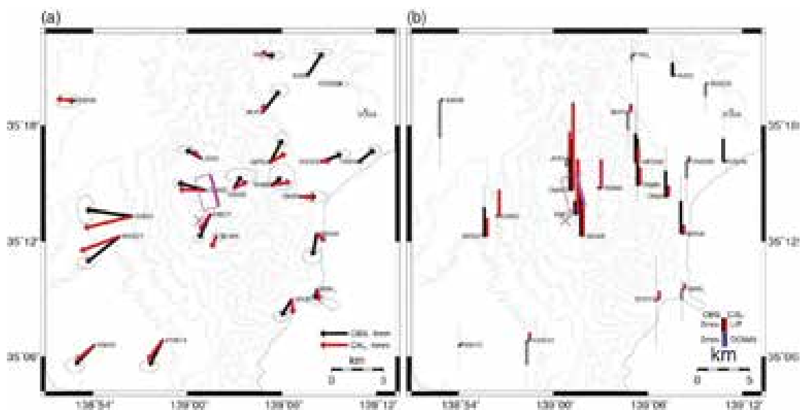
図 45. 道家ほか (2019) 34) による、活動初期における変位ベクトルおよびモデルによるシミュレーション結果。(a) 水平変位、(b) 上下変位。ベクトルは、2019 年 2 月 19 日～ 28 日と 2019 年 5 月 23 日～ 6 月 1 日のそれぞれの平均値の差分で示している。ピンク色の×印が茂木モデル、矩形が開口クラックモデル (太線が上端) の位置を示す。パラメータの詳細は道家ほか (2019) 34) を参照。
