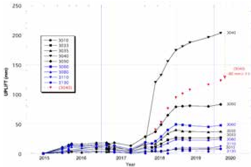
図 39. 主な水準点の標高の時間変化。2017 年 10 月以降は隆起傾向がみられ、地下の圧力源の急膨張が推定されていたが、2018 年 12 月以降は多くの観測点ではほぼ停止状態である。BM3040 は硫黄山西側噴気孔近傍の県道沿いに位置し、2018 年 4 月 20 日からの硫黄山西側噴気の活発化に伴い局所的に約 8cm の隆起がみられ、その後も局所的に変化が大きいため、圧力源解析では使用していない。
