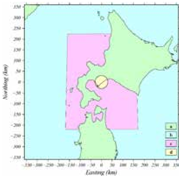
図 47. 倶多楽火山の 3 次元比抵抗構造モデルの計算範囲と使用した陸域および海域の地形データの種類と範囲。倶多楽湖の中心付近を原点とする座標系で、中心から±360km の範囲をモデル化した。a:ETOP01 22) (陸域)、b:ETOP01 (海域)、c:日本海洋データセンターの J-EGG500 35) 、d:陸域：国土地理院の基盤地図情報 10m メッシュ数値標高モデル、海域：日本水路協会発行の M7006 (津軽海峡東部)。
