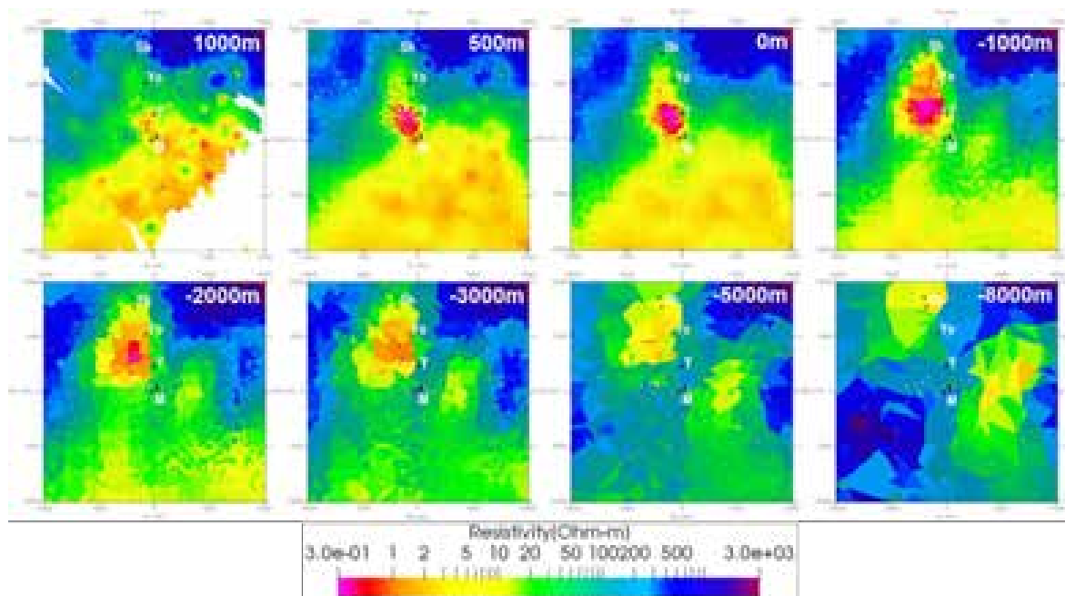
図 23. 草津白根火山周辺の暫定比抵抗構造モデル。標高 1000m、500m、0m、-1000m、-2000m、-3000m、-5000m、-8000 m の水平断面を示す。Sh: 志賀山・鉢山、Yo: 横手山、Y: 湯釜、M: 本白根山。白点は MT 観測点。
