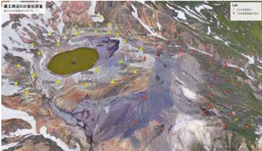
図 31. (上) 令和 2-3 年度観測予定点図(赤二重丸)。楕円 A,B はアクセスが困難とみられる地域。黄二重丸は平成 26 年度に実施した観測点。(下) 観測予定点の鳥観図。赤ピンマーク：令和 2-3 年度観測予定点、黄ピンマーク：平成 26 年度に実施した観測点。人的アクセス可能な限界範囲まで観測点を配置した。
